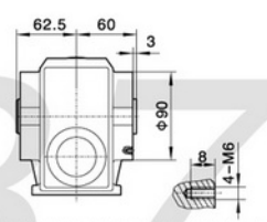
S..37R17
