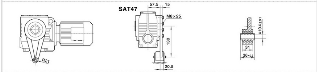
S..S47
