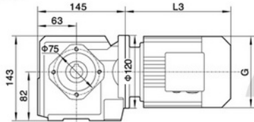
SA37
