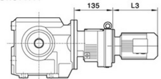
S..S37
