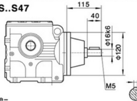
S..S47
