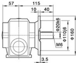
SF37/φ160
