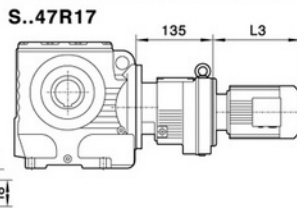
S..47R17
